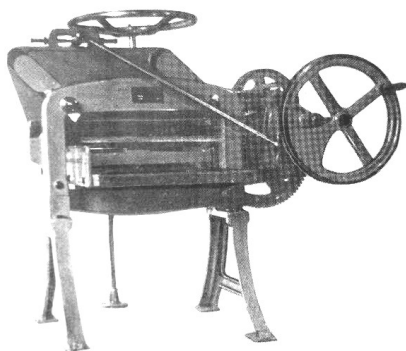
Паперорізальна одноножова машина моделі БР -7, ручна, малоформатна. Така машина випускалась в кінці 30-х років.
