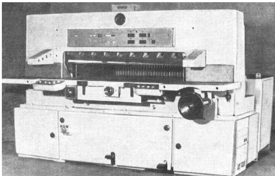
Паперорізальна одноножова машина з програмовим управлінням, магнітною стрічкою і цифровою індикацією БР-39 ПУ, випускалась у середині восьмидесятих.
